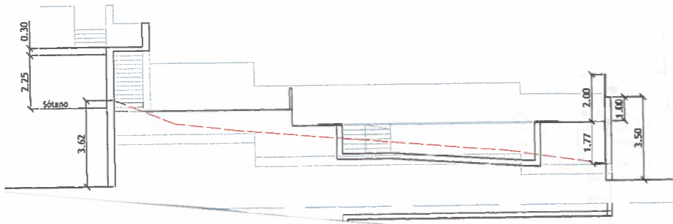
Img 7. Sección recogida en el proyecto.
